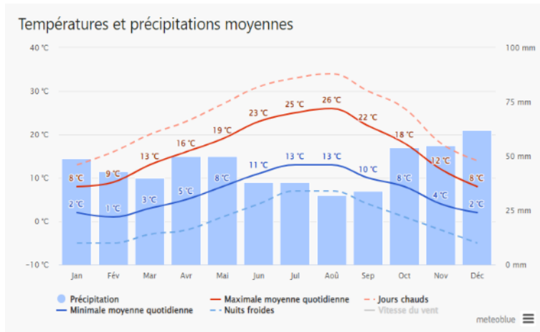
Températures et précipitations moyennes (station météorologique Chartres)
