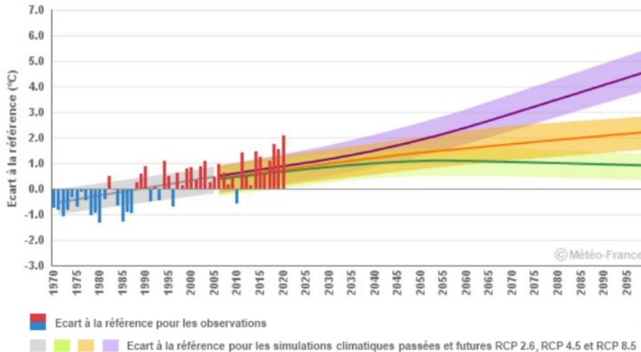
Température moyenne annuelle en Centre-Val de Loire : écart à la référence 1976-2005. Observations et simulations climatiques pour trois scénarios d'évolution RCP 2.6, 4.5, et 8.5
