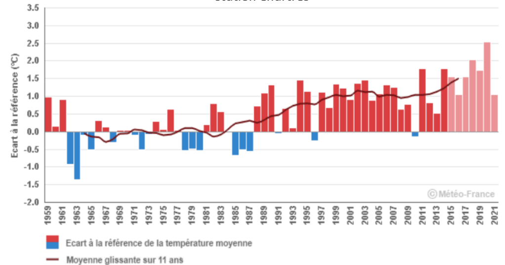
Températures moyennes annuelles : écart à la référence 1961-1990, station Chartres
