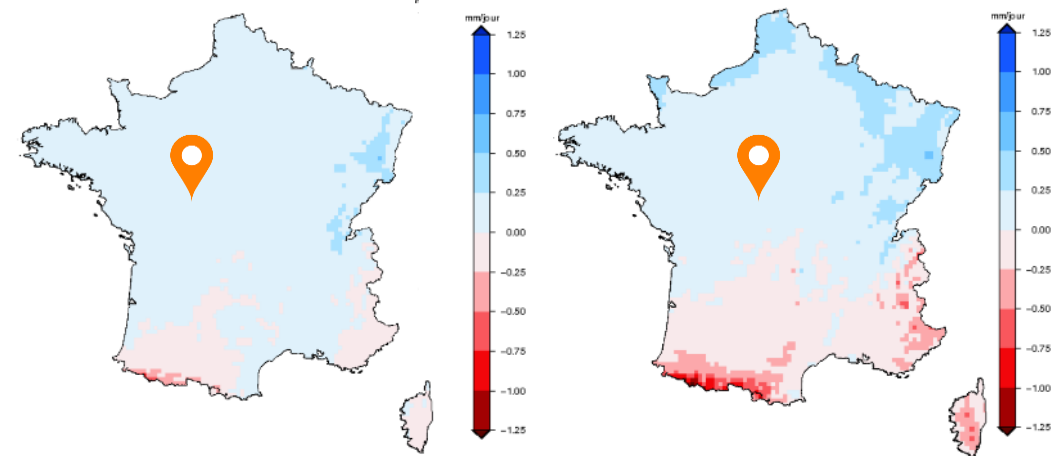
Cumul annuel de précipitation : écart entre la période considérée et la période de référence pour horizon moyen (2041-2070) carte de gauche et pour horizon lointain (2071-2100) carte de droite , pour un scénario sans politique climatique (RCP 8.5)
