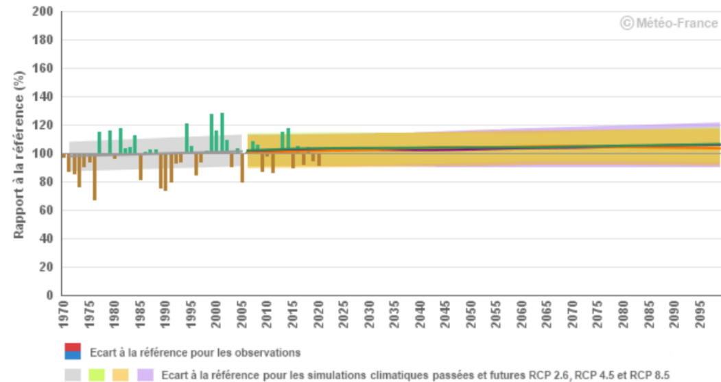
Cumul annuel de précipitations en Centre-Val de Loire : rapport à la référence 1976-2005. Observations et simulations climatiques pour deux scénarios d'évolutions RCP 2.6, 4.5 et 8.5
