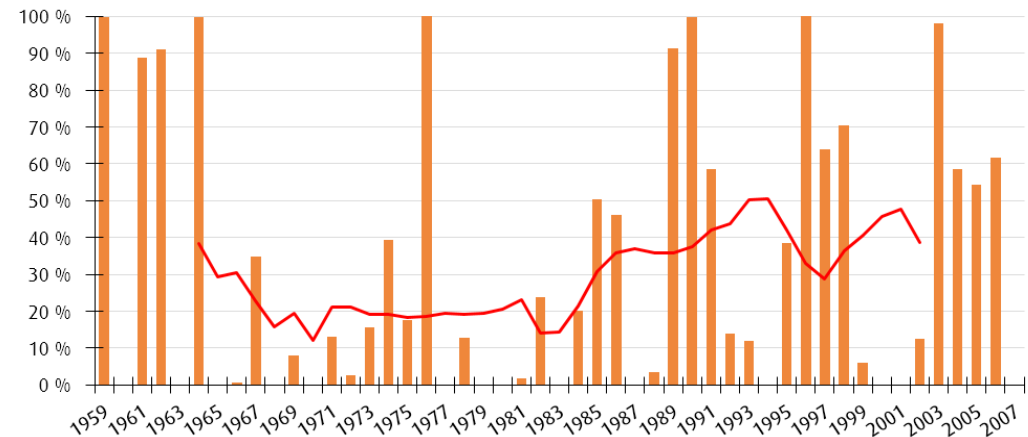
Pourcentage annuel de la surface régionale touchée par des conditions propices aux départs de feux de forêts (IFM > 20 pendant plus d'un mois), région Centre-Val de Loire
