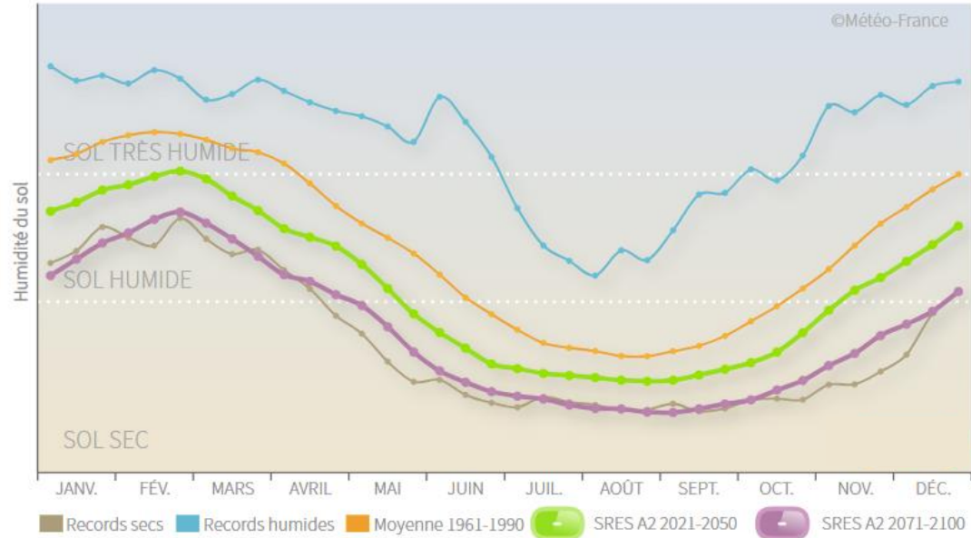
Cycle annuel d'humidité du sol (moyenne 1961-1990), records et simulations climatiques pour deux horizons temporels (scénario d'évolution SRES A2), Centre-Val de Loire
