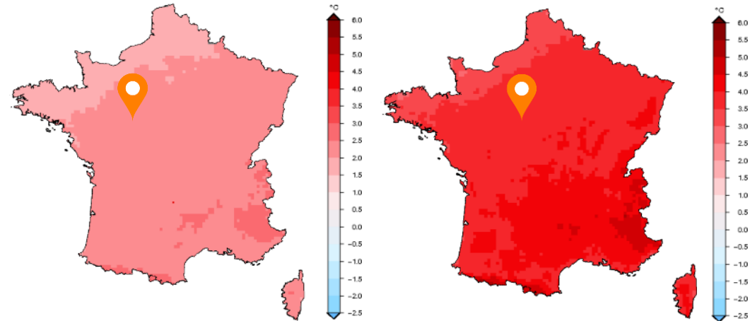
Anomalie de température moyenne quotidienne : écart entre la période considérée et la période de référence pour horizon moyen (2041-2070) carte de gauche et pour horizon lointain (2071-2100) carte de droite , pour un scénario sans politique climatique (RCP 8.5)
